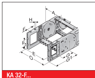
КА 32-F...
